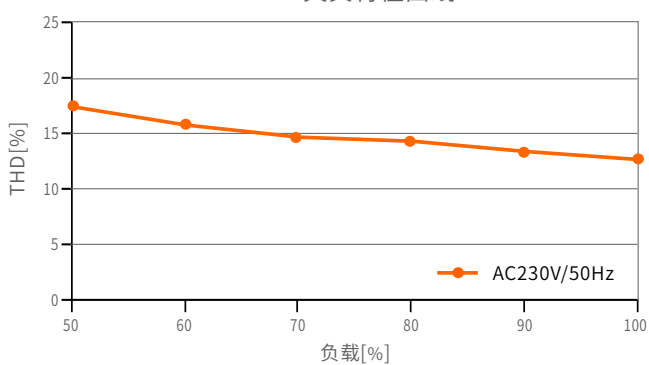
THD失真特征曲线
