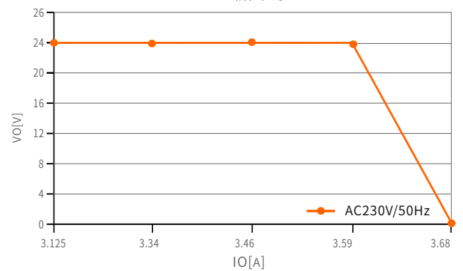
过载曲线
