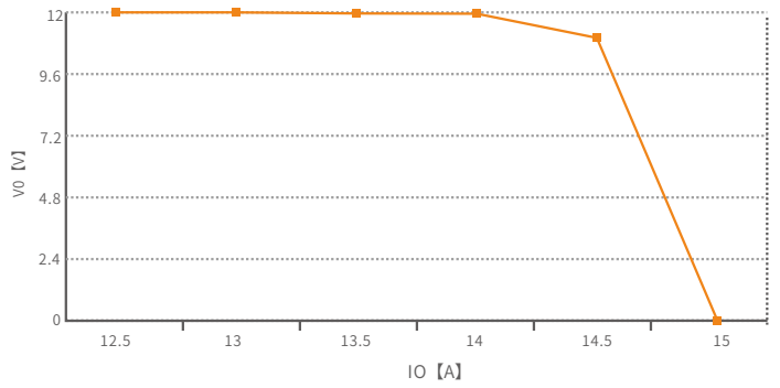
过载曲线
