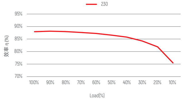
效率曲线
