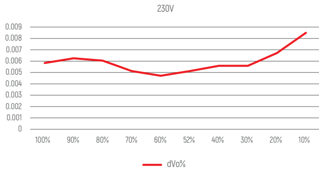
负载调整率曲线
